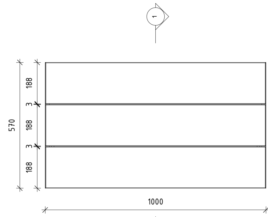
Ansichten 1:10
