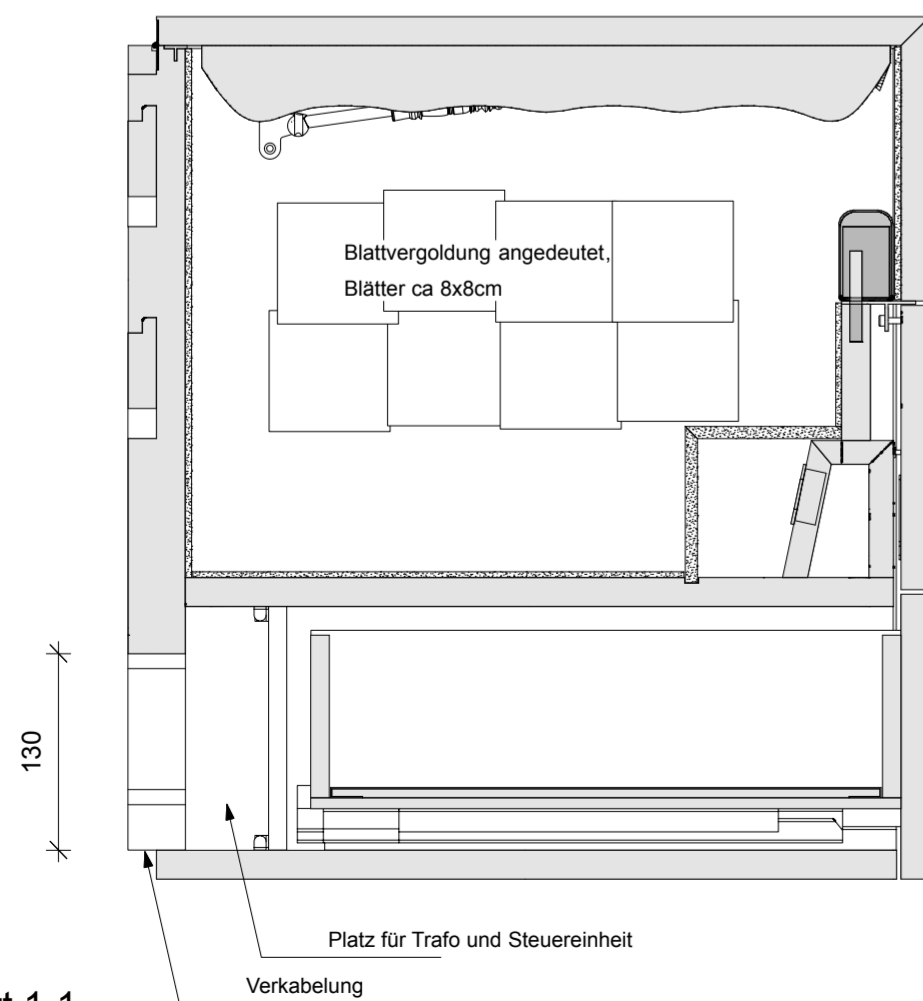
Schnitt 1-1 1:5
