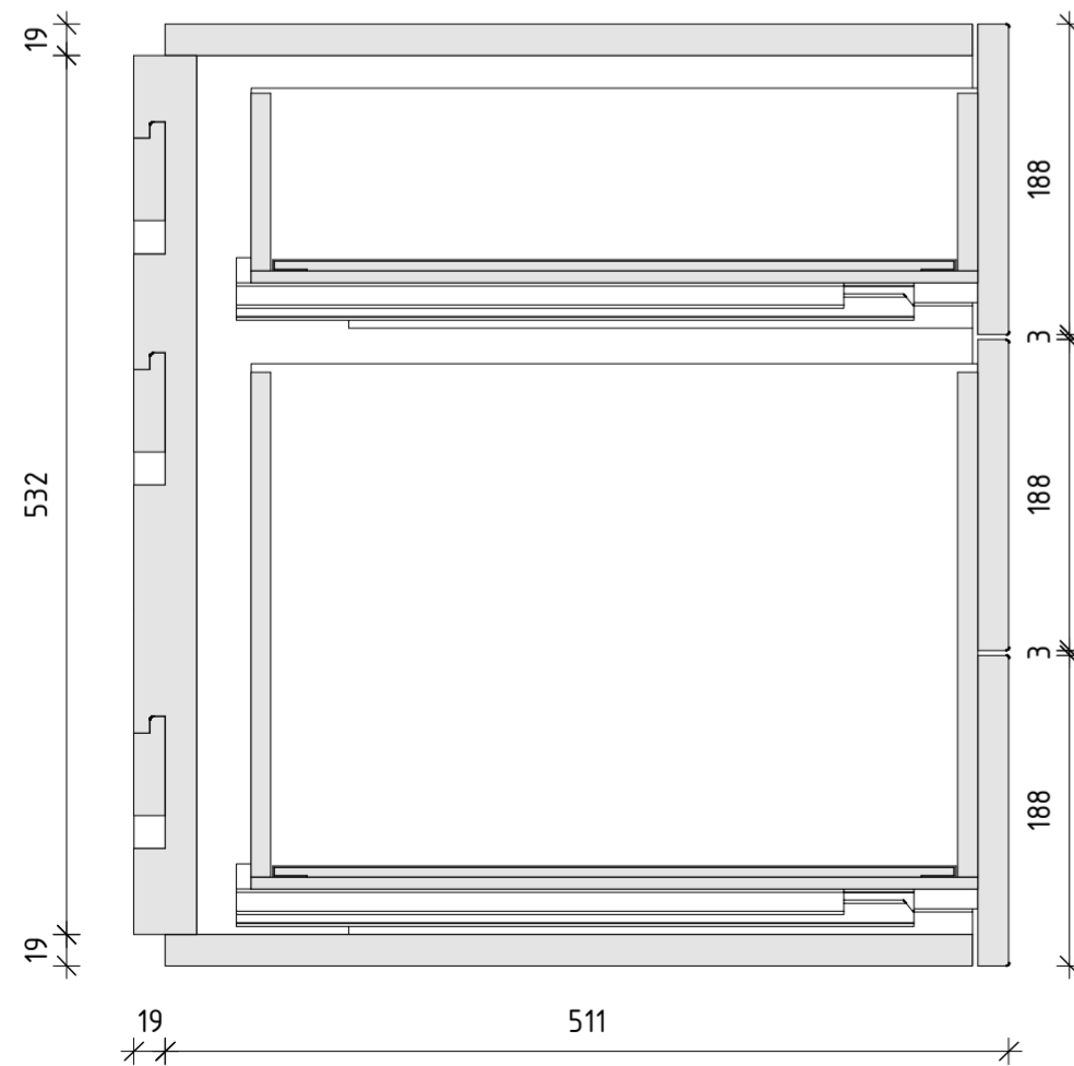
Schnitt 1-1 1:5
