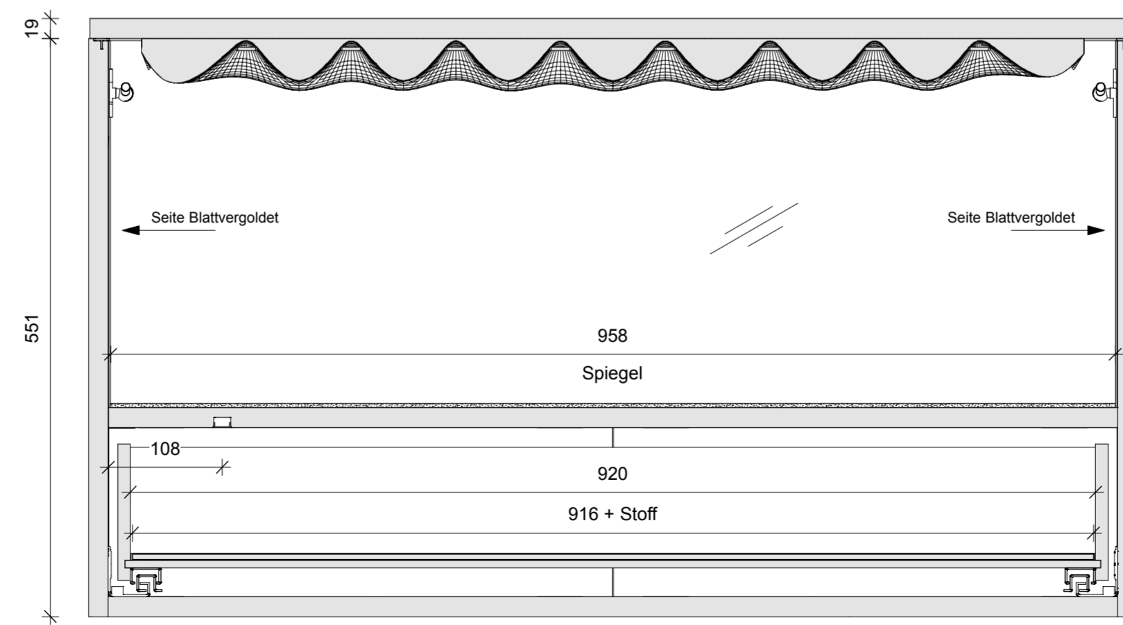
Schnitt 2-2 1:5
