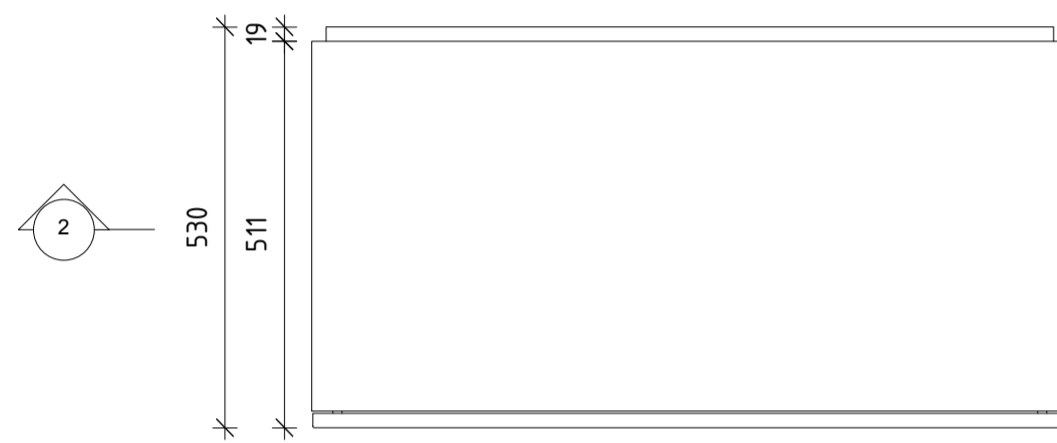
Ansichten 1:10
